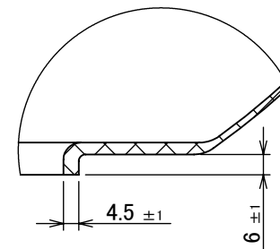
詳細図 A スケール 1 : 2
