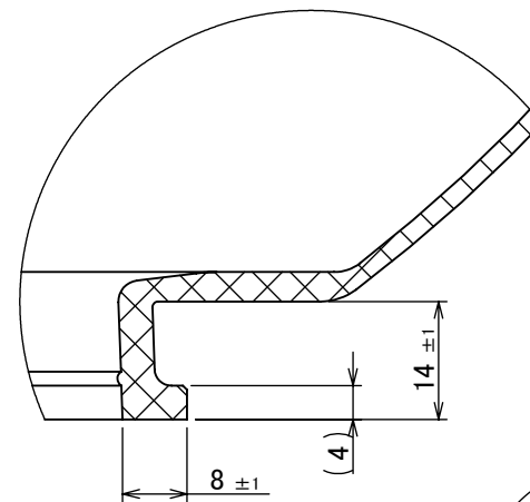
詳細図 A スケール 1:1
