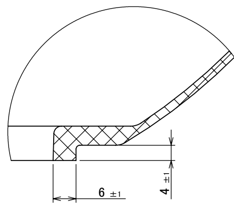
詳細図 A スケール 1:1
