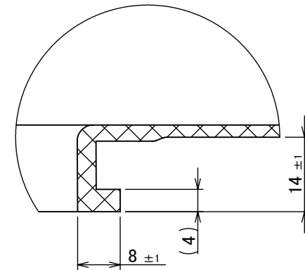
詳細図 A スケール 1 : 1
