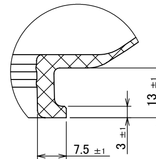
詳細図 A スケール 1 : 1
