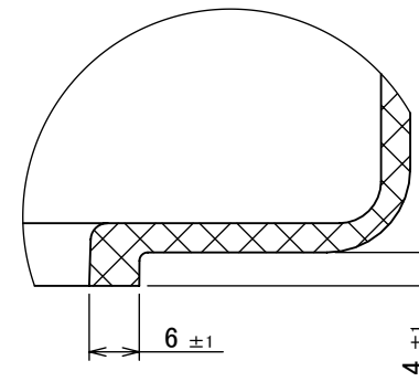
詳細図 A スケール 1 : 1
