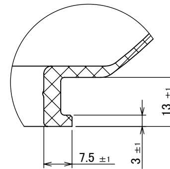
詳細図 A スケール 1 : 1
