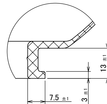
詳細図 A スケール 1:1
