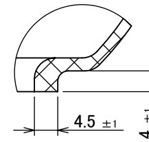
詳細図 A スケール 1:1
