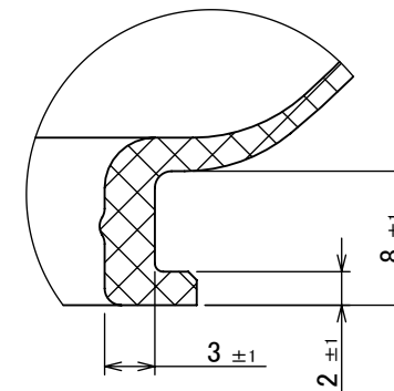
詳細図 A スケール 2 : 1
