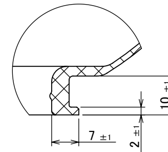
詳細図 A スケール 1:1
