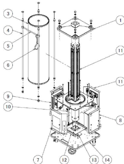
分解図
